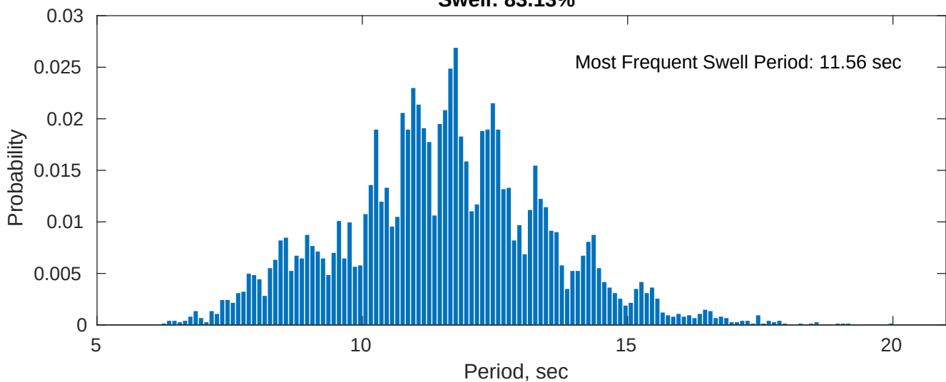
Swell: 83.13%
